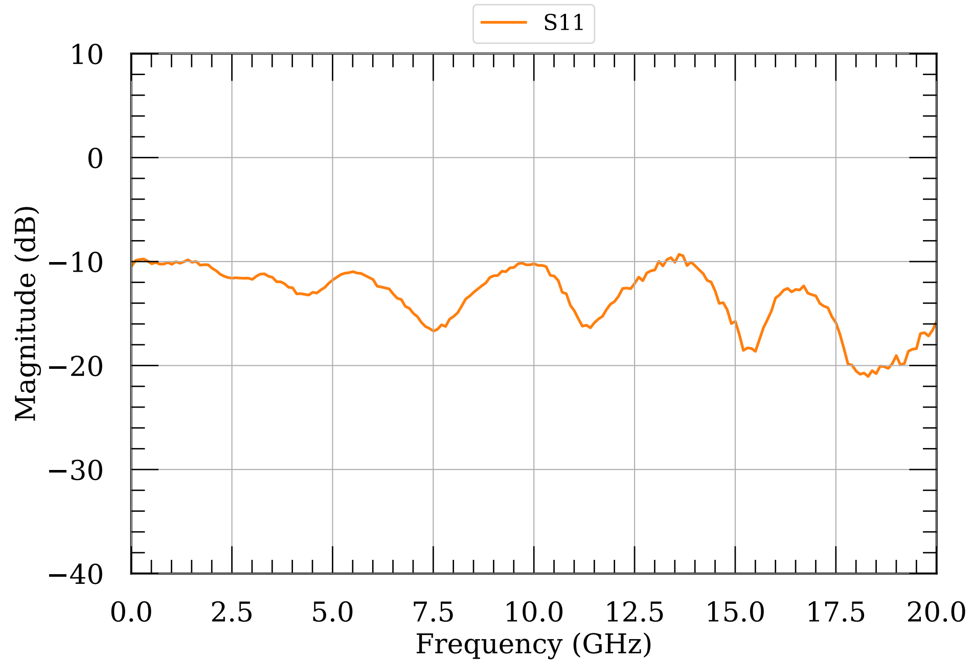
LNA S-params module054v2
